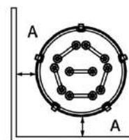
Distance de sécurité Poêle Tower
